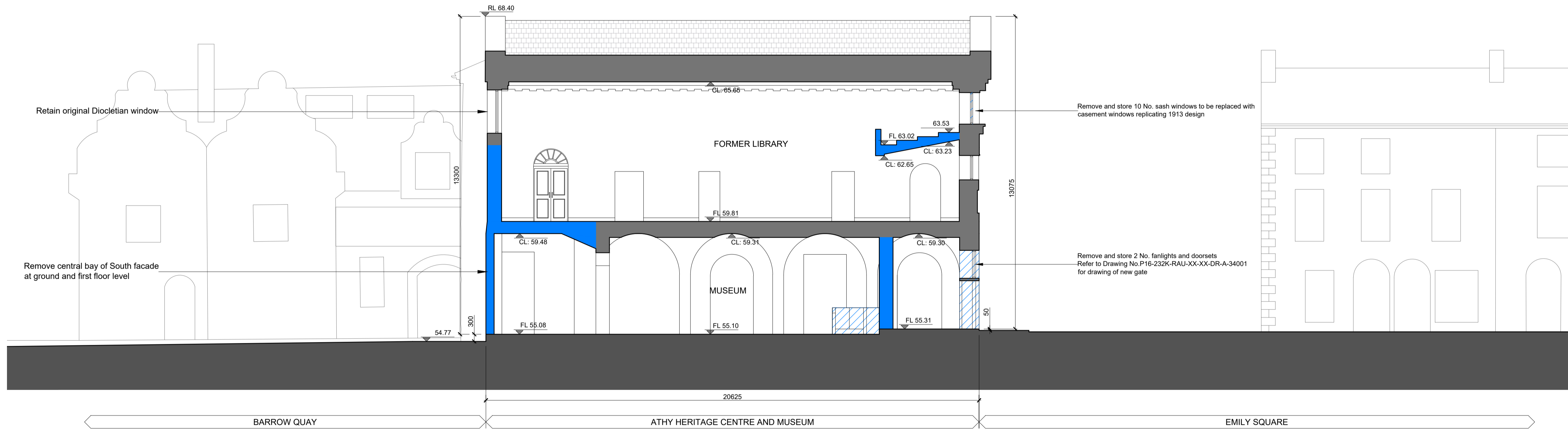
1 EXISTING SECTION C-C 1:100@A1 1:200@A3
